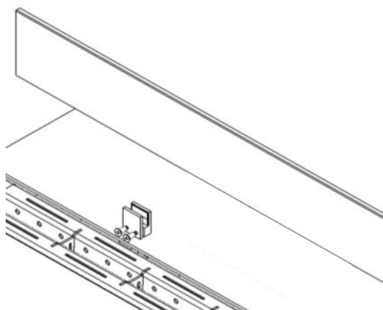
Illustration 2. Réglage du verre frontal.
