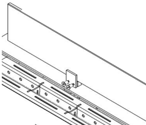
Illustration 3. Dernière étape de l'installation du verre frontal (serrer les supports)
