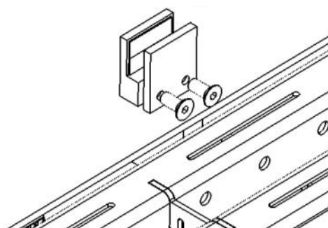
Illustration 1. Dévisser les vis du support
