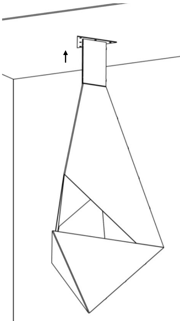
Illustration 4 - Fixation au plafond
