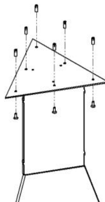
Illustration 4 - Fixation au plafond
