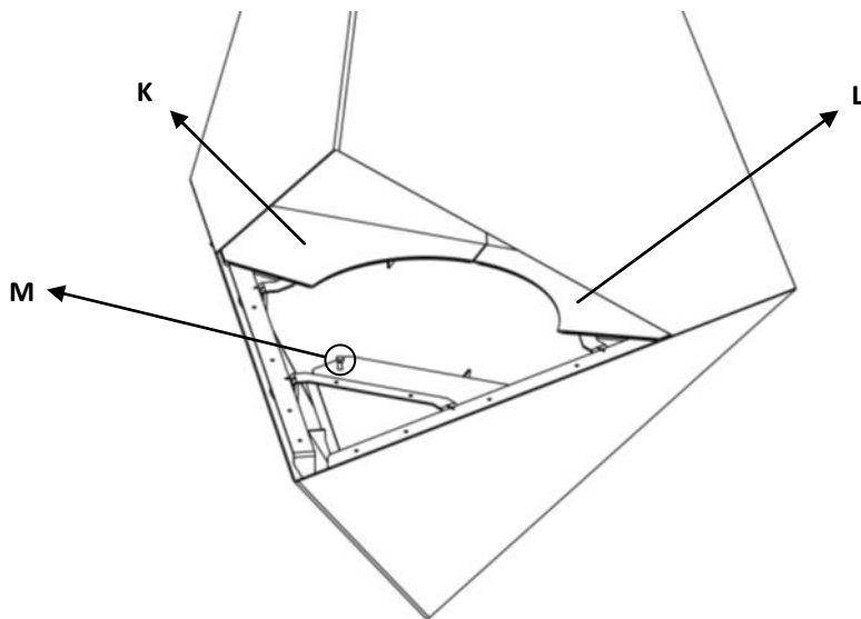
Illustration 6 - Cheminée avec les plaques décoratives préalablement installées
