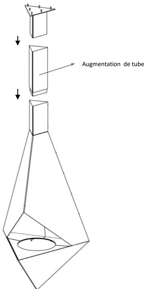
Figura 13— Montage de l'augmentation de tube.
