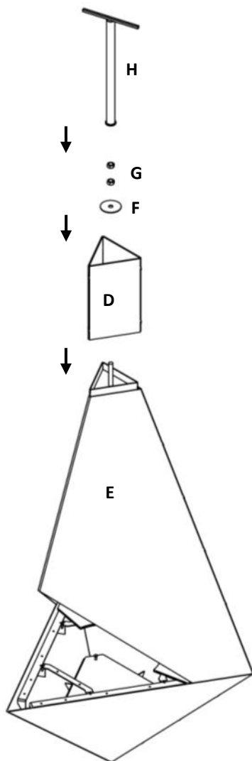
Illustration 1 — Représentation du montage
