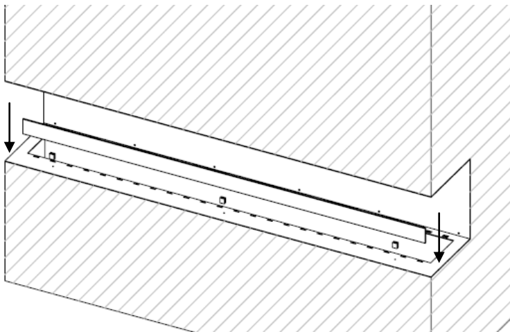
Figure 3 —Installation de e verre protecteur
