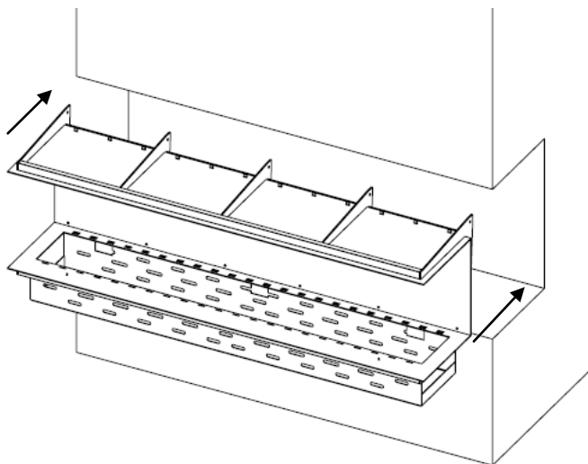
Figure 1 —Placement la cheminée dans la niche préalablement effectué
